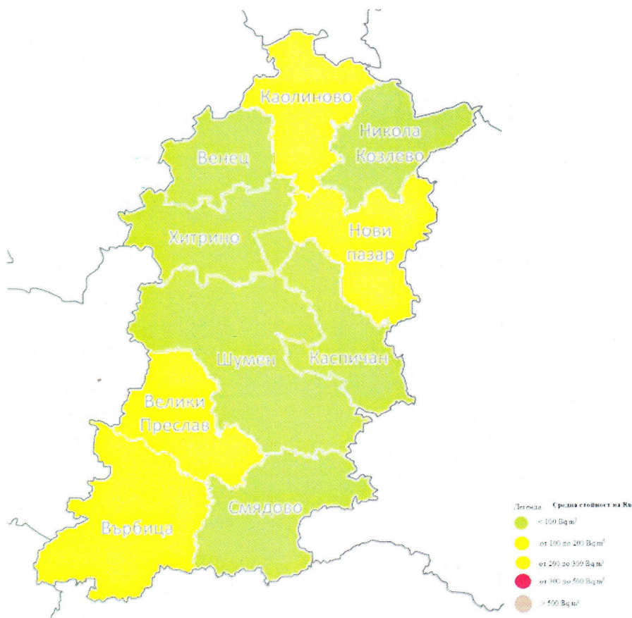
Карта - Средната стойност на концентрацията на радон във жилища по общини за област Шумен
